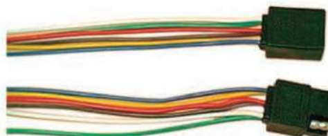
ENCHUFES DE 6 CONTACTO COD. 15.2507 HEMBRE 10 Unid. COD. 15.2508 MACHO 10 Unid.
