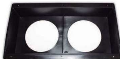
COD. 028.0245 MARCO PLASTICO PARA FAROL ALTO: 18.5CM LARGO: 33CM PROFUNDIDAD: 5.5CM DIAMETRO CIRCULAR: 11.5CM
